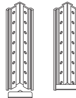
Рис. 2. Установка подпятника на стойку.
