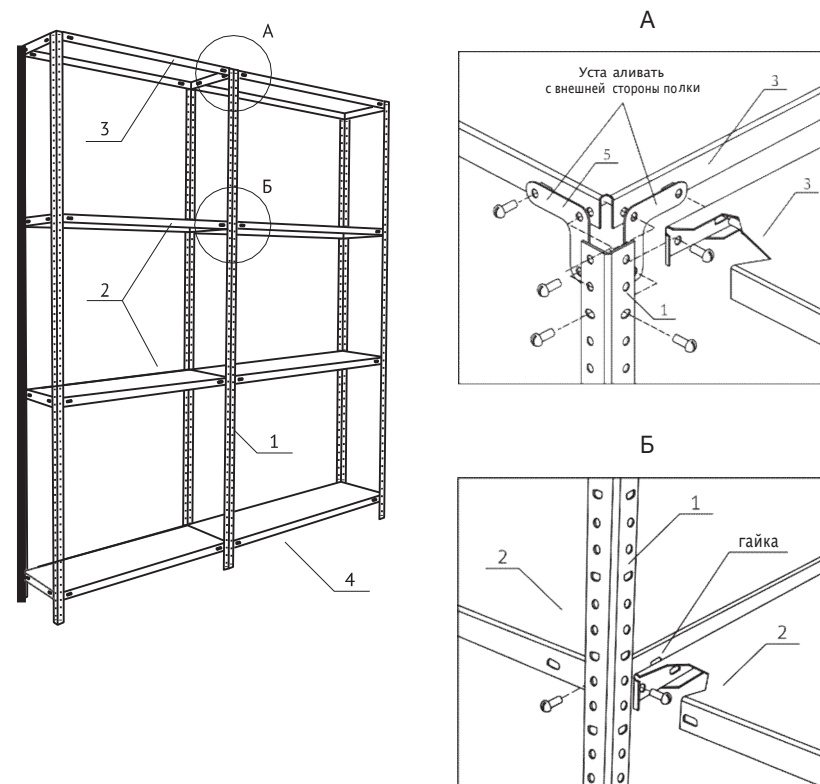
Рис. 4. Сборка стеллажа серии СТ ленточным способом.
