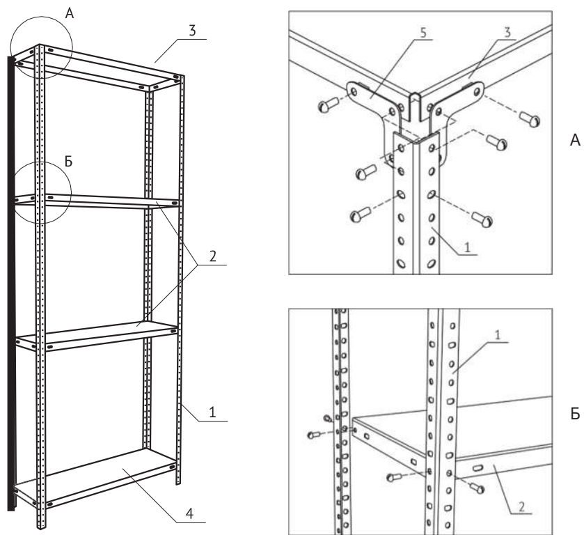
Рис. 3. Сборка одной секции стеллажа СТ.
